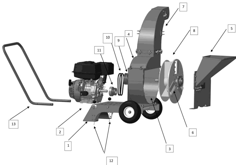
Рис. 3 – Устройство садового измельчителя
